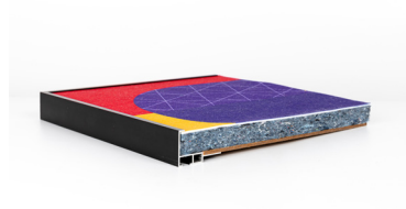
Querschnitt AcousticPro basic
